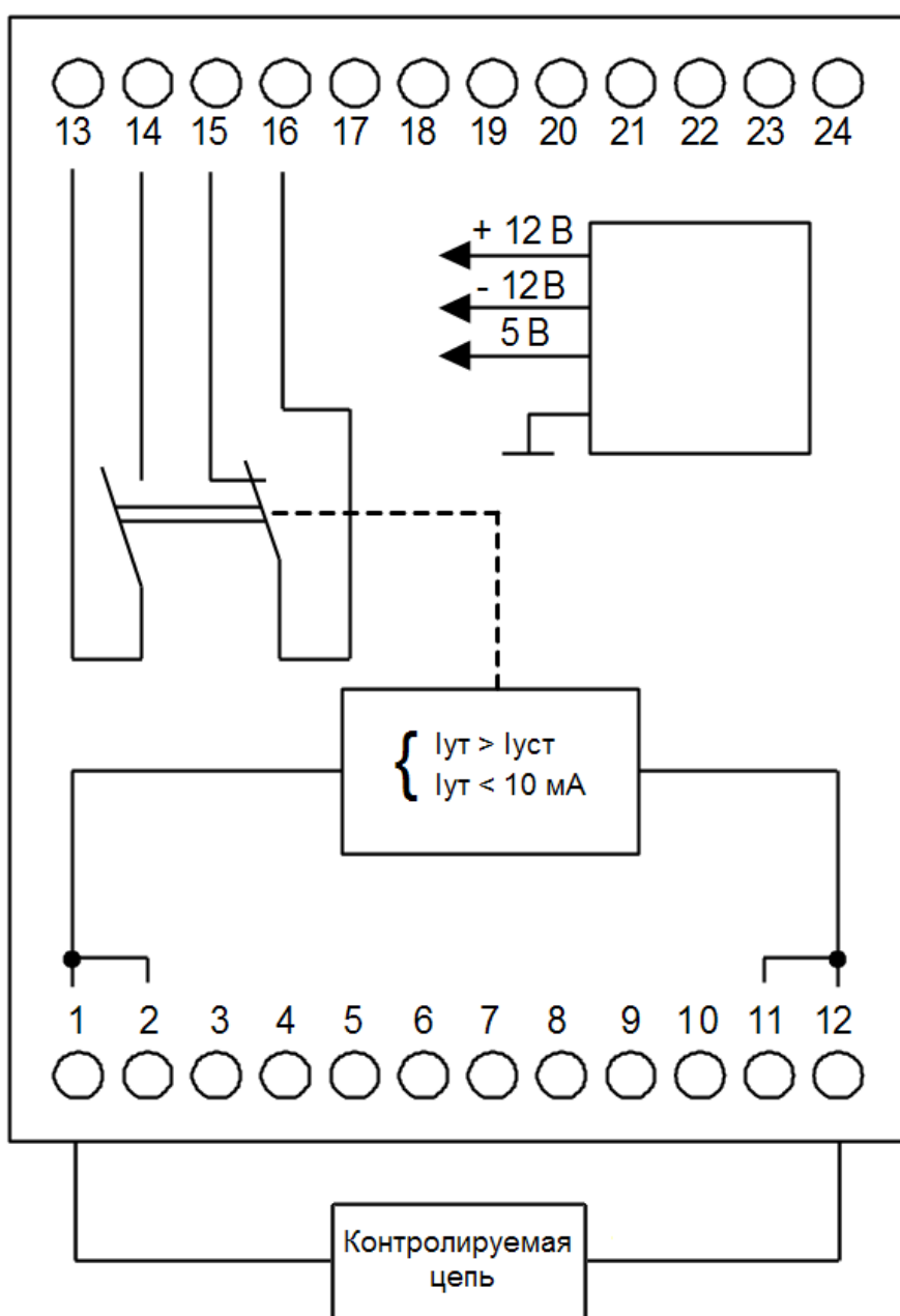
Рисунок 3. Схемы подключения и расположения выводов реле
