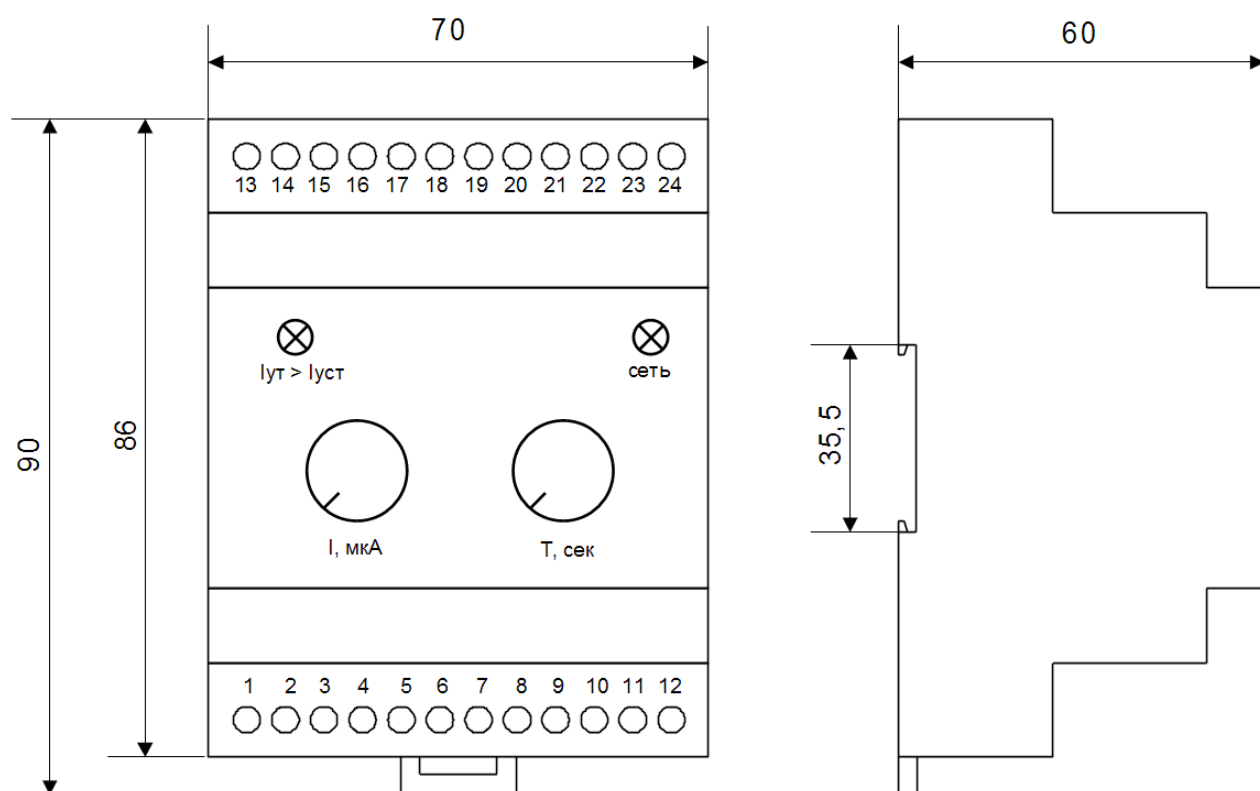
Рисунок 2. Реле РК-32
