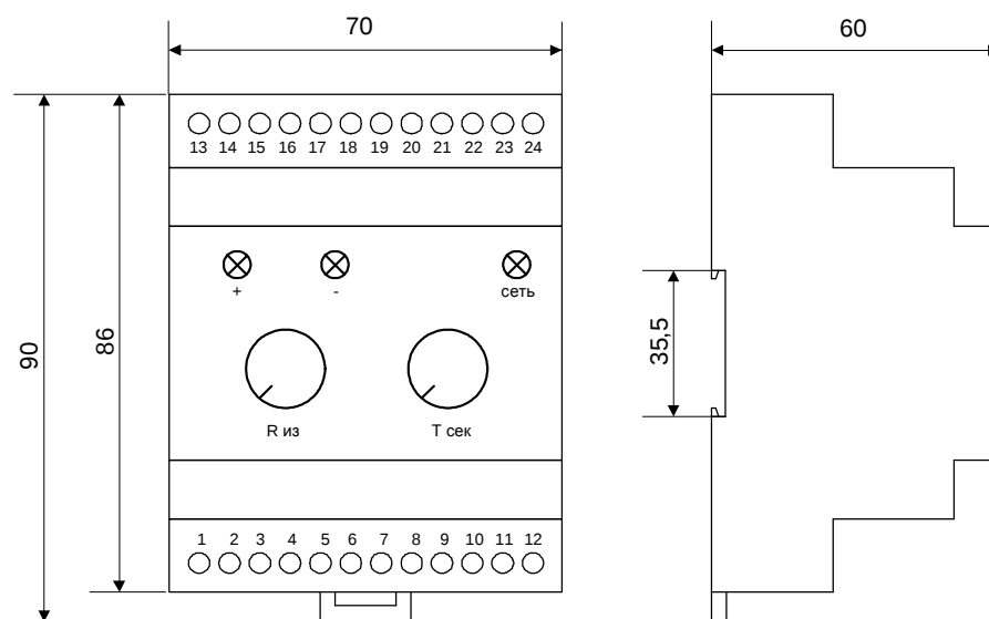
Рисунок 2 Реле РК-30
