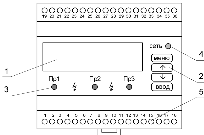
Рисунок 3 – Передняя панель реле
