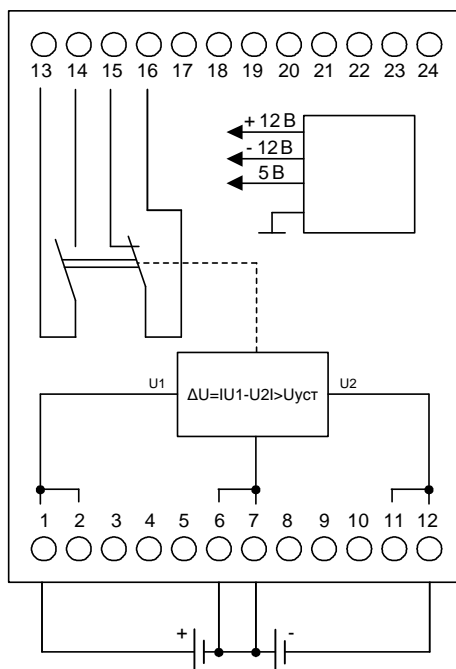
Рисунок 3 Схемы подключения и расположения выводов реле
